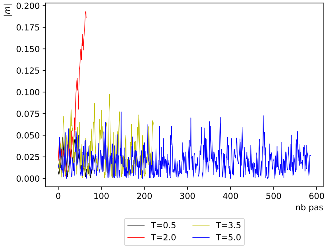
Evolution de l'Aimantation suivant un pas de MonteCorlo pour différentes températures
